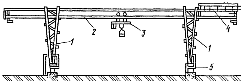
Рис. 10. Кран-перегрузчик трубчатой конструкции
