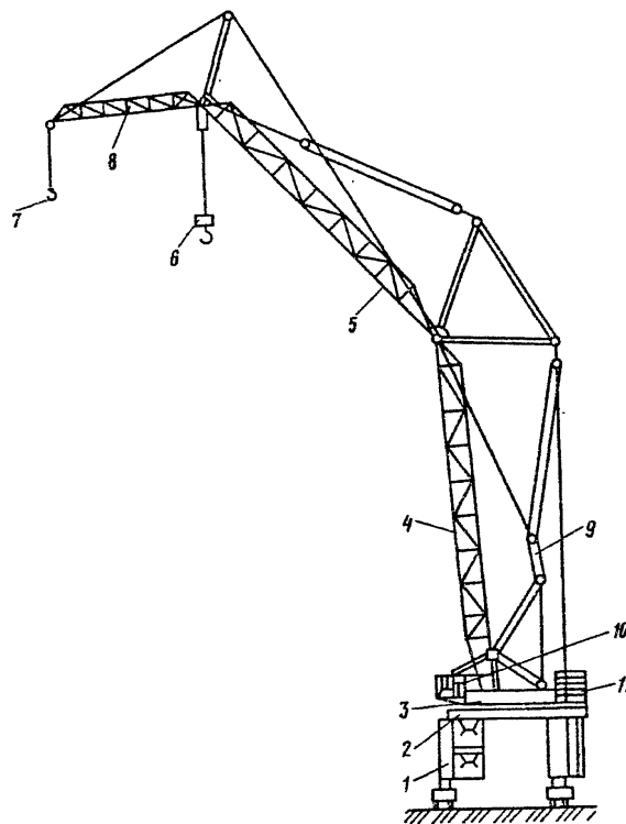
Рис. 8. Кран башенно-стреловой СКР-3500ЭМ
