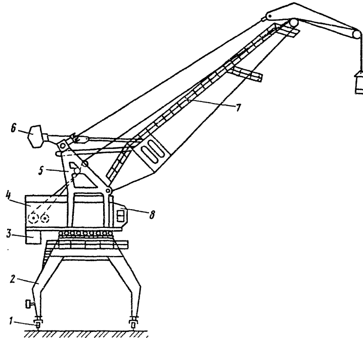
Рис. 5. Кран порталный
