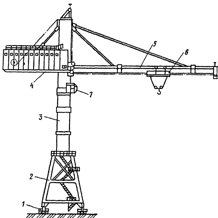
Рис. 7. Кран башенный трубчатой конструкции
