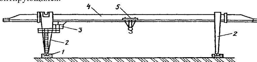
Рис. 3. Кран козловой самомонтирующийся
